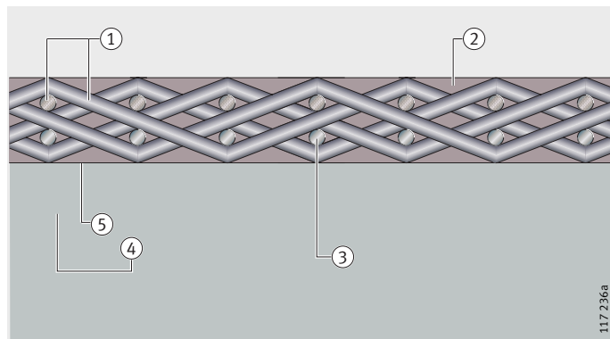
Figura 1 ELGOGLIDE ® – sezione
