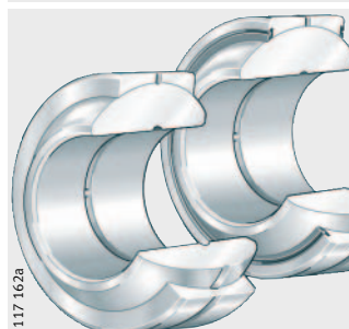
GE..-HO-2RS
